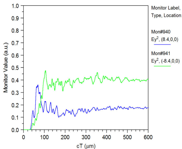
شکل 6. توان نوری برای حالت A=1, B=1
