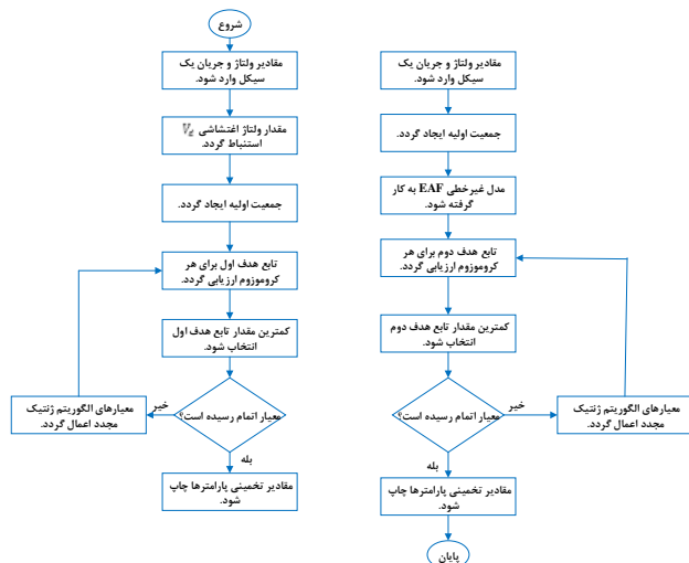
شکل (۱): اعمال الگوریتم ژنتیک بر حل مسأله‌ی بهینه‌سازی
