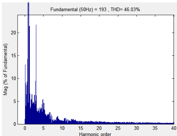
شکل (۹): طیف فرکانسی پاسخ جریان کوره قوس الکتریکی با پارامترهای تخمینی و SVC
