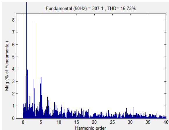
شکل (۸): طیف فرکانسی پاسخ ولتاژ کوره قوس الکتریکی با پارامترهای تخمینی و SVC
