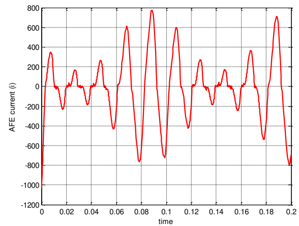
شکل (۳): پاسخ جریان کوره قوس الکتریکی در ساختار مرسوم
