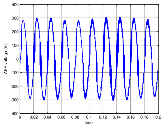
شکل (۶): پاسخ ولتاژ کوره قوس الکتریکی با پارامترهای تخمینی و SVC
