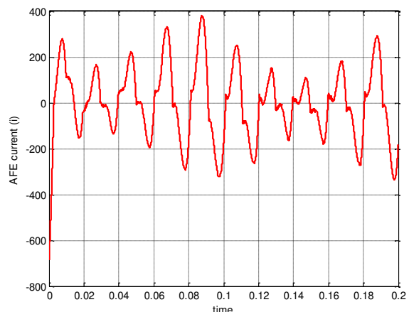
شکل (۷): پاسخ جریان کوره قوس الکتریکی با پارامترهای تخمینی و SVC با دقت در پاسخ شکل موج ولتاژ کوره قوس با به کارگیری پارامترهای تخمینی و SVC، شکل موج حاصل به حالت سینوسی ایده آل نزدیک تر بوده و در نتیجه ضریب اعوجاج هارمونیک کمتری دارد. با دقت در شکل ۷ مشاهده می شود که پاسخ جریان تغییر چندانی نسبت به پاسخ های جریان قبلی از حیث ضریب اعوجاج هارمونیک ندارد و تنها اندازه ی این جریان هارمونیک کاهش یافته است.
