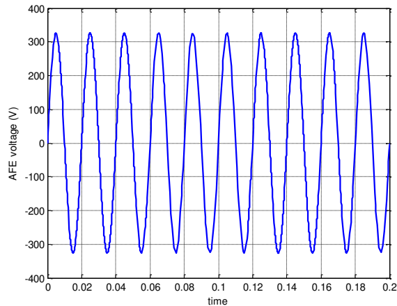
شکل (۲): پاسخ ولتاژ کوره قوس الکتریکی در ساختار مرسوم
