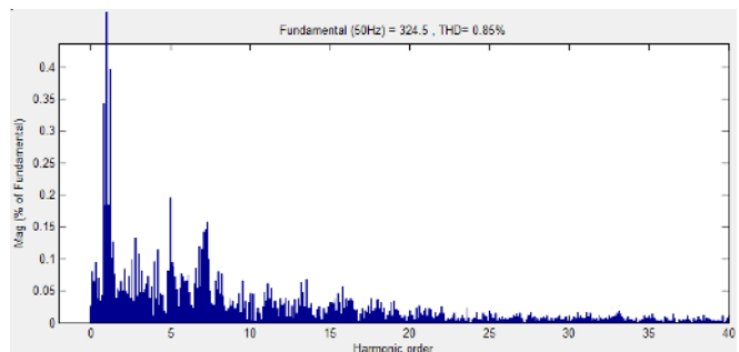
شکل (۴): طیف فرکانسی پاسخ جریان کوره قوس الکتریکی در ساختار
