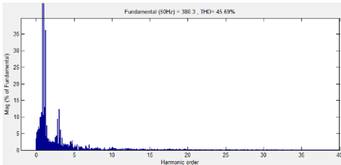
شکل (۵): طیف فرکانسی پاسخ جریان کوره قوس الکتریکی در ساختار مرسوم
